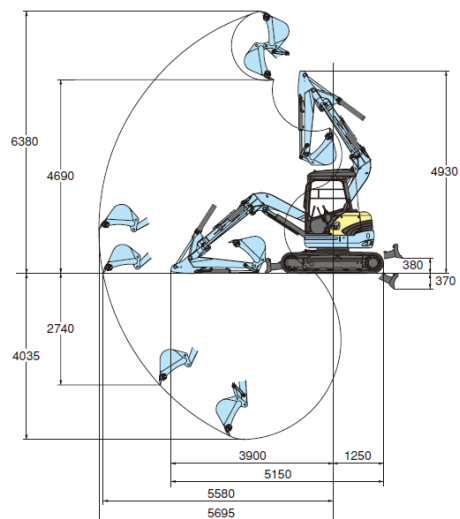
■作業範囲・外観寸法図 単位 (mm)
