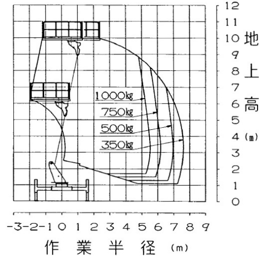
■作業範囲図 (アウトリガ最大張出時)
