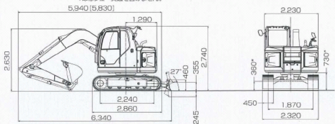
■全体図(単位: mm) アーム1.71m、バケット0.28m 3 装着時。[ ]内はドーザ前向き時の値です。 *印はシュー突起を含みません。
