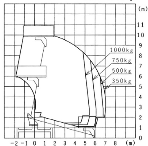
アウトリガ張出幅 最大 最大積載荷重1000kg
