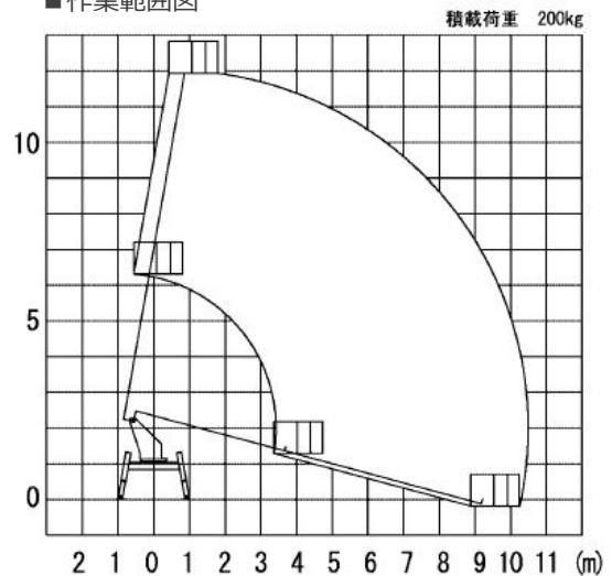
■作業範囲図
