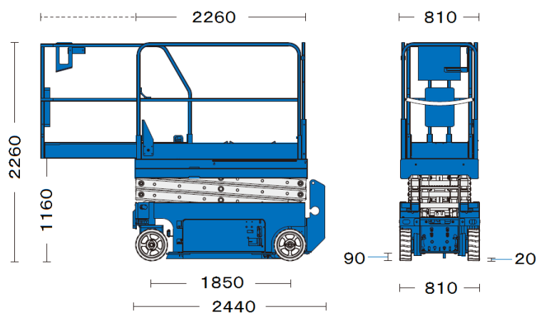
■寸法図 単位: mm
