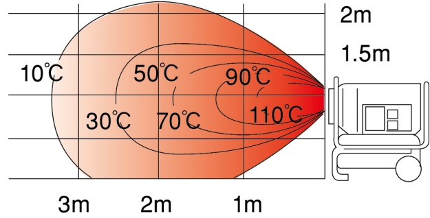
●温度分布図（上昇温度0℃基準）
