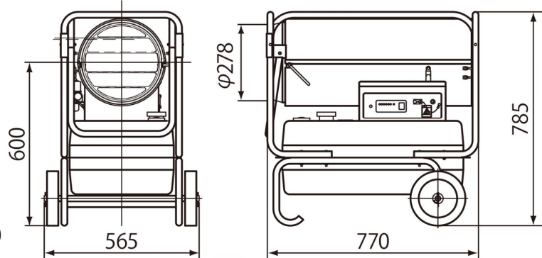
■外形図 単位: mm
