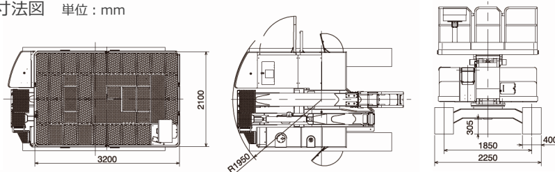
■ 寸法図 単位：mm
