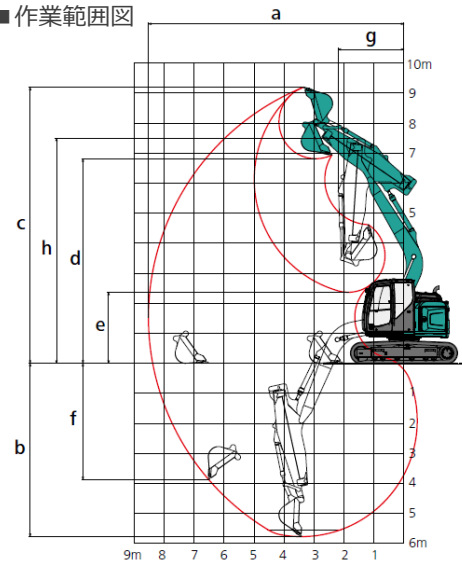
■作業範囲図
