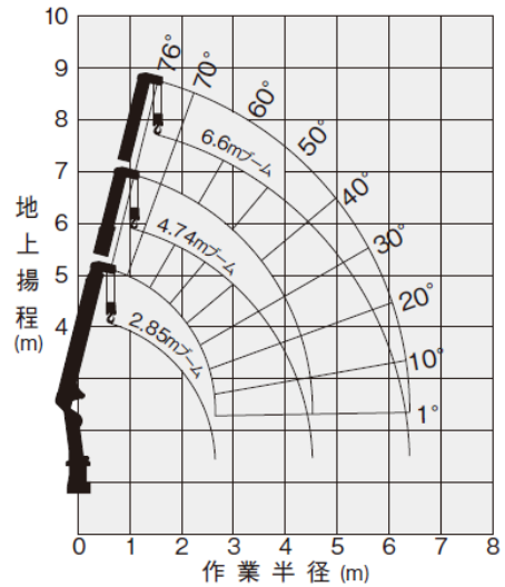
■作業半径・揚程図
