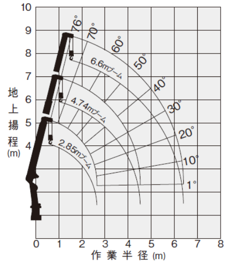
■作業半径・揚程図
