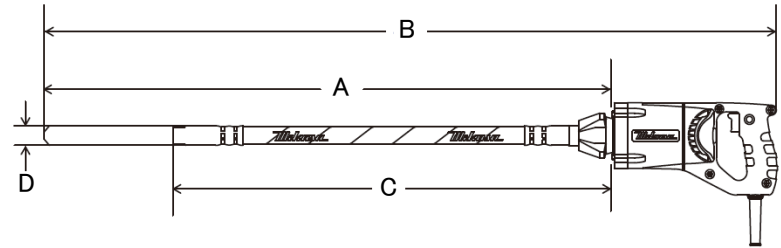
■寸法図
