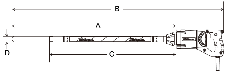
■寸法図
