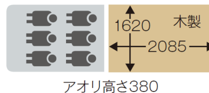
■荷台寸法 単位mm
