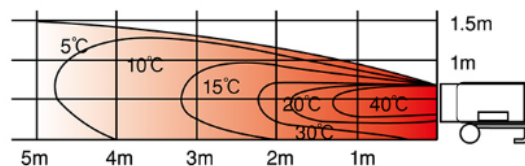
●温度分布図(上昇温度0℃基準)
