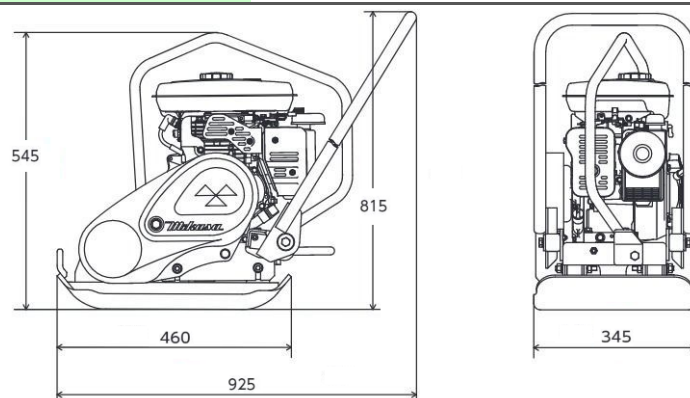
■外形寸法図 単位：mm
