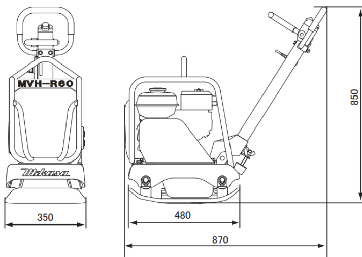
■ 外観寸法図 単位：mm
