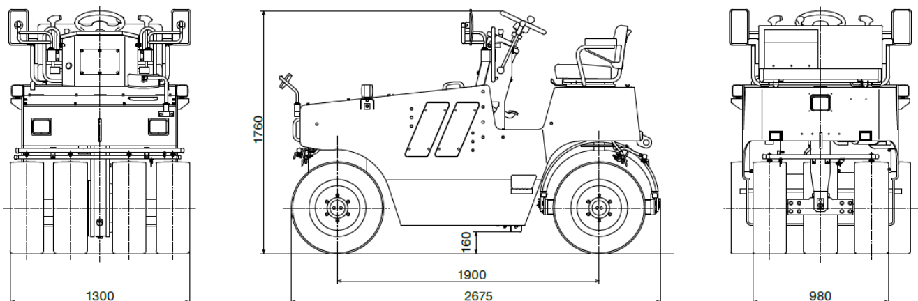
■寸法図 単位：mm
