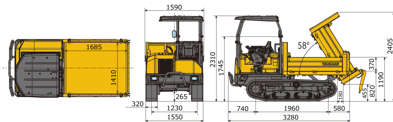
■外形寸法図 単位 : mm
