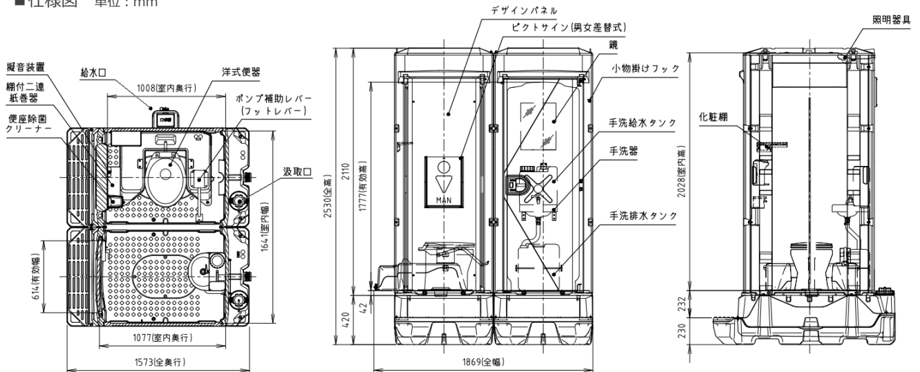
■仕様図 単位：mm
