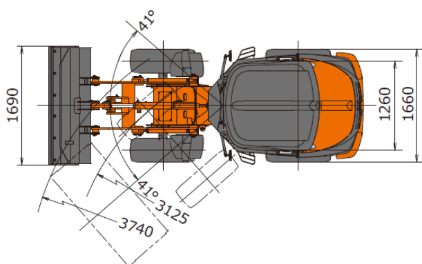
■寸法図 単位: mm
