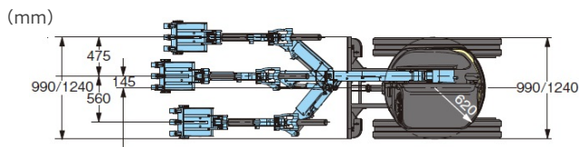
■ 寸法・作業範囲図
